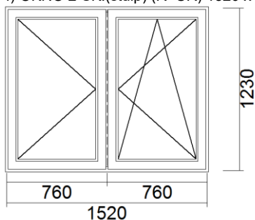
4) OKNO 2-SK.(štulp) (R+UR) 1520 x 1230
