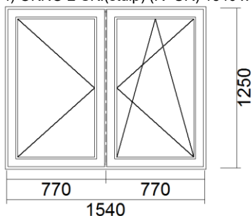
4) OKNO 2-SK.(štulp) (R+UR) 1540 x 1250
