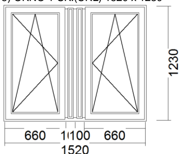
5) OKNO 1-SK.(URL) 1520 x 1230
